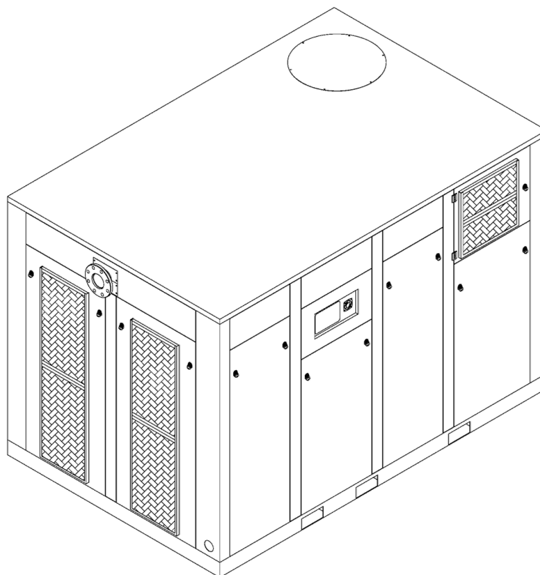
Рисунок 1 – Общий вид компрессорной станции ЗИФ-СВЭ ШМЧ (ЗИФ-СВЭ ШМЧ-Р)
