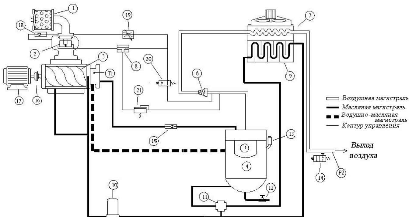
Рисунок 8 – Схема комбинированная функциональная станции компрессорной электрической ЗИФ-СВЭ ШМЧ (ЗИФ-СВЭ ШМЧ-Р)
