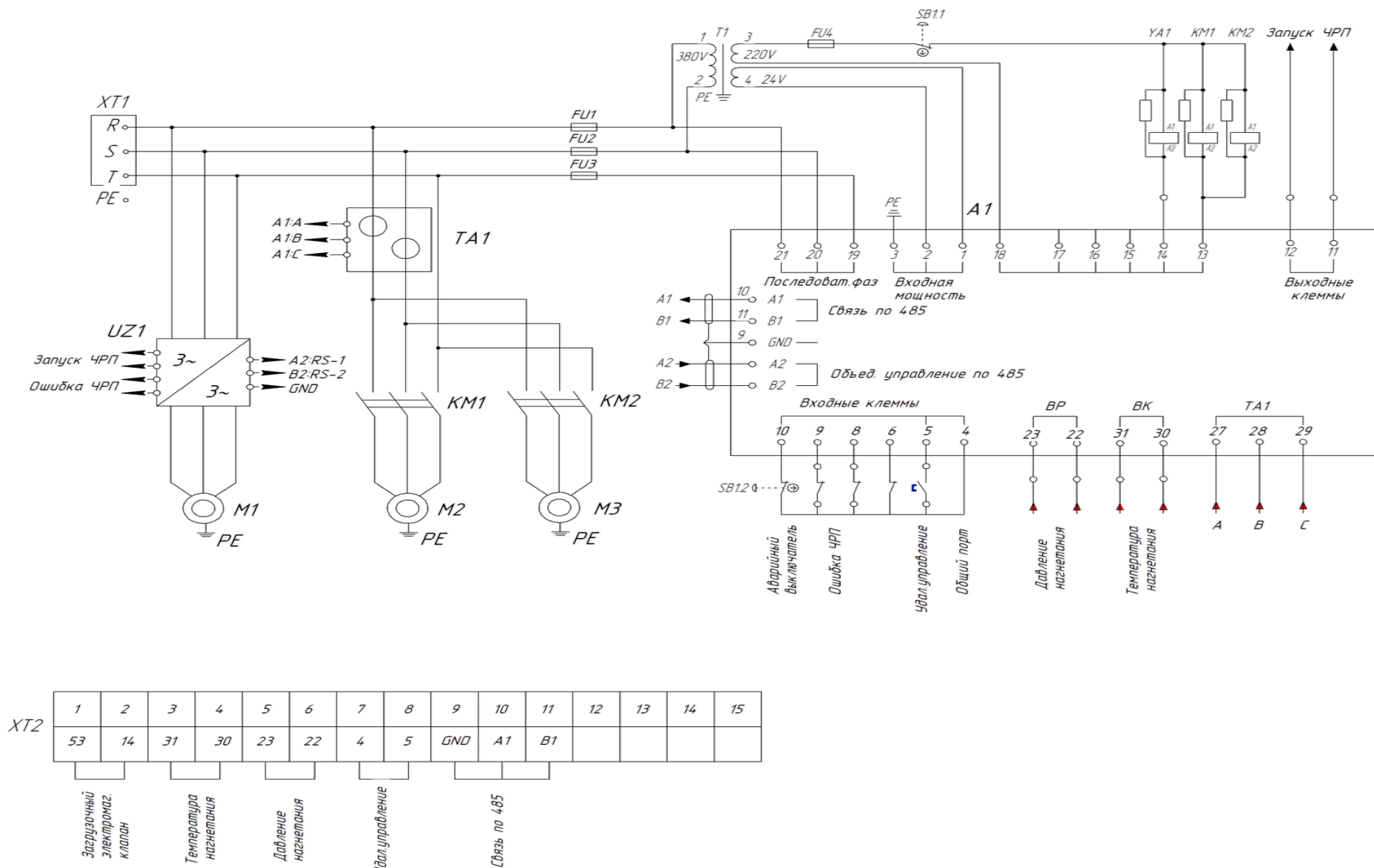
Рисунок Б.1 – Схема электрическая принципиальная станции компрессорной электрической ЗИФ-СВЭ ШМЧ (ЗИФ-СВЭ ШМЧ-Р)
