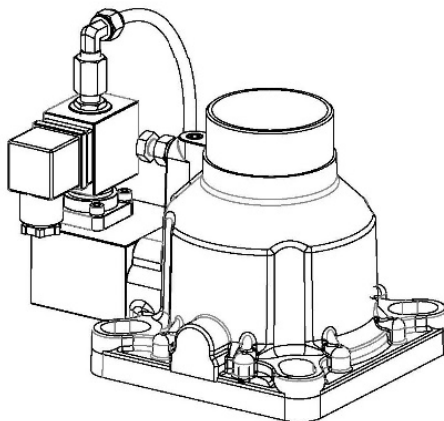
Рисунок 19 – Впускной клапан
