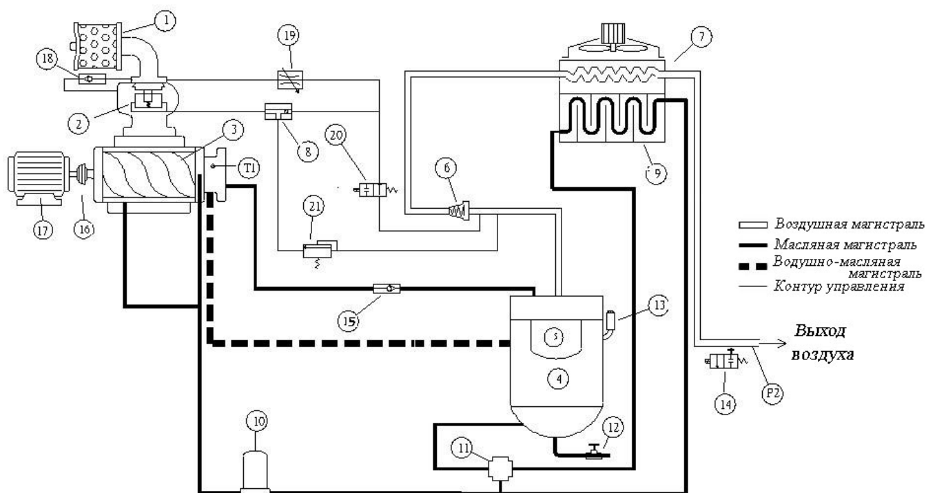
Рисунок 9 – Схема комбинированная функциональная станции компрессорной электрической ЗИФ-СВЭ ШМЧ
