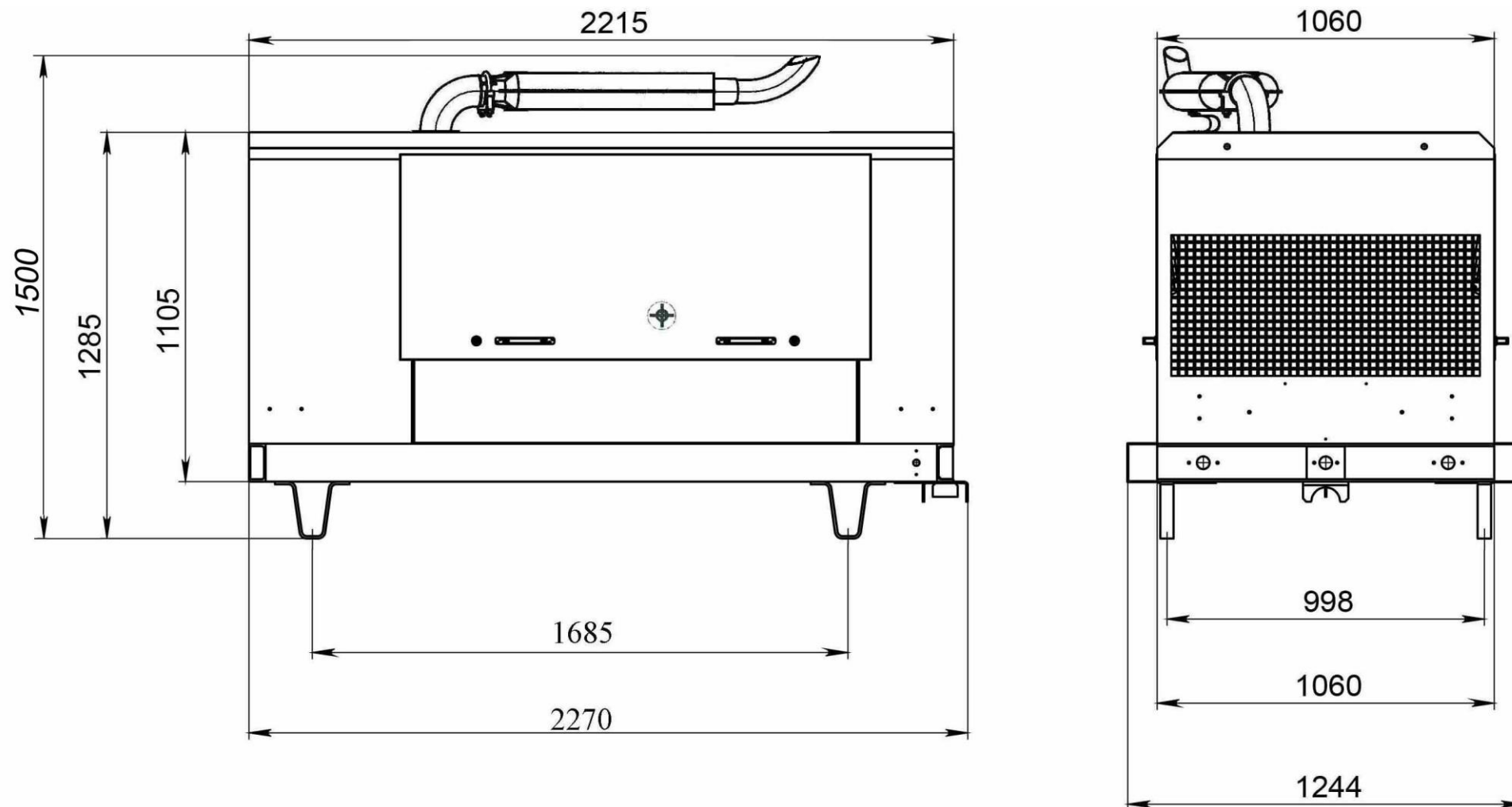
Рисунок В.1 - Габаритный чертеж компрессорной станции ЗИФ-ПВ8/1,0 (АРМ9-50-06). Исполнение на раме.
