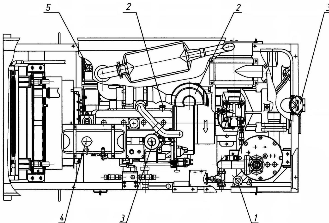
Рисунок В.13 - Схема заправки компрессорной станции ЗИФ-ПВ 8/1,0 (APM9-50-06) ( см. приложение А )
