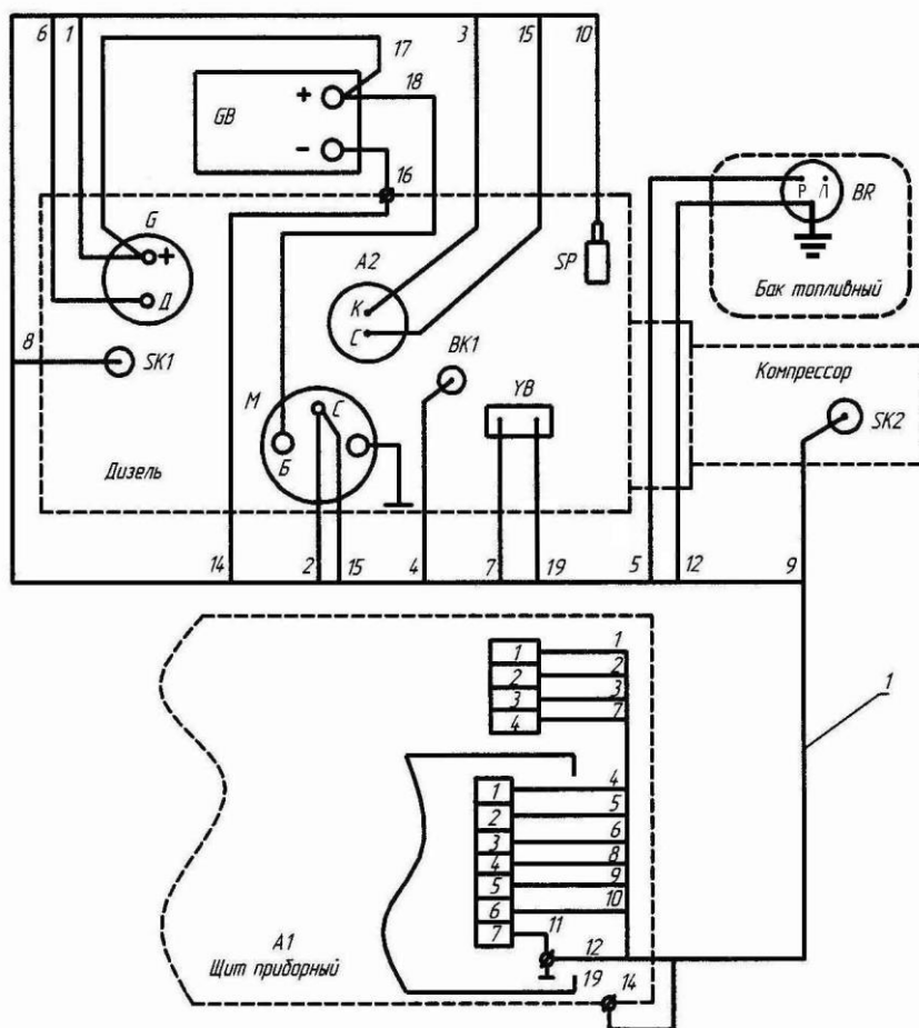
Рисунок В.11 – Схема электромонтажная компрессорной станции ЗИФ-ПВ 8/1,0 (APM9-50-06)
